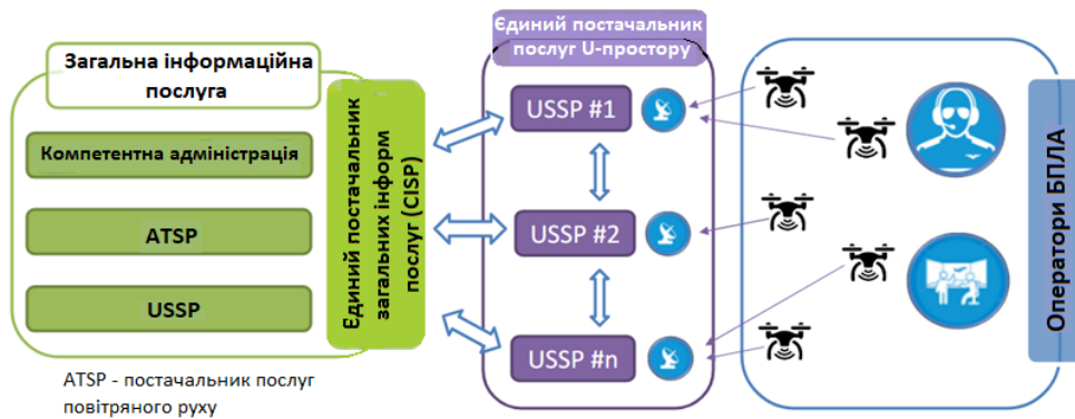
Рис.1 Архітектура U-простору [9]
