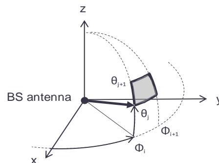
Рис.7 Виділення фрагменту (площадки) у фронті електромагнітної хвилі
