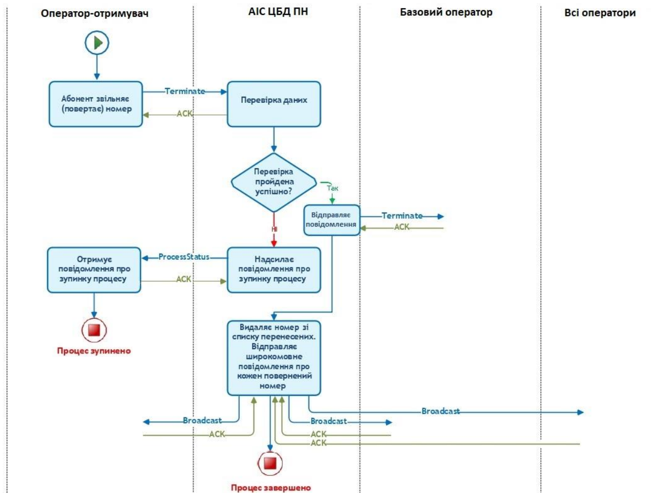
Рис. 5. Схема процесу повернення номера
